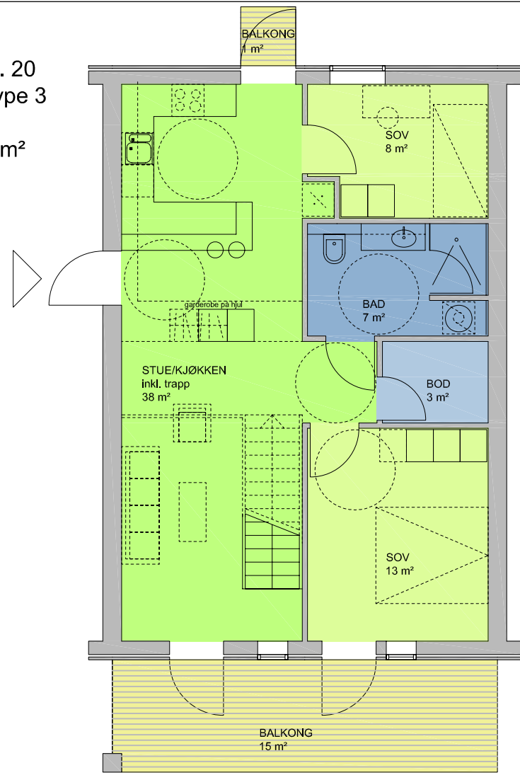
4.etasje
